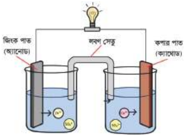
চিত্র ৮.১৬: গ্যালভানিক কোষের সাহায্যে বিদ্যুৎ শক্তি উৎপাদন
