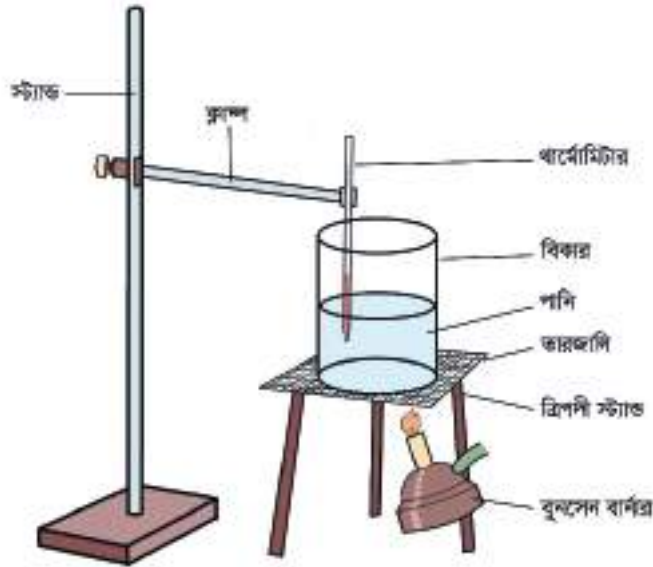
চিত্র ২.০৮: পানির স্ফুটনাঙ্ক নির্ণয়
