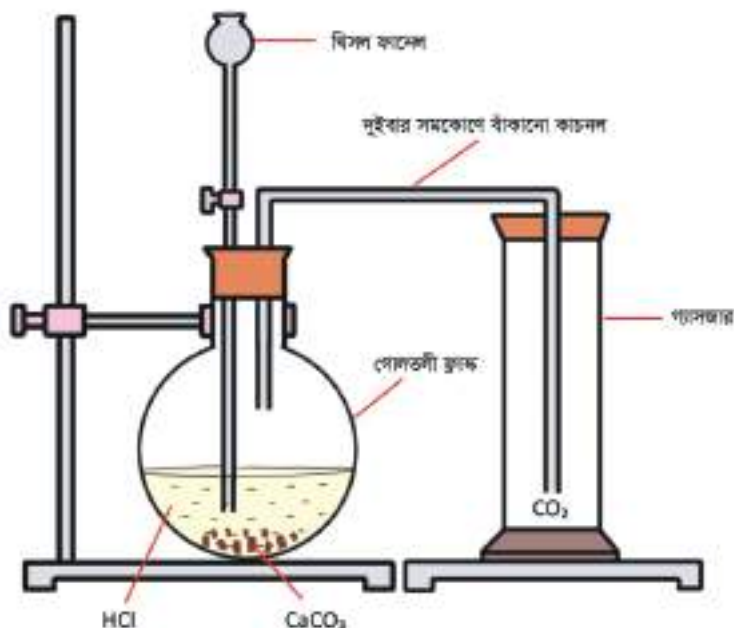
চিত্র ৪.০৩: কার্বন ডাই-অক্সাইড প্রস্তুতকরণ
