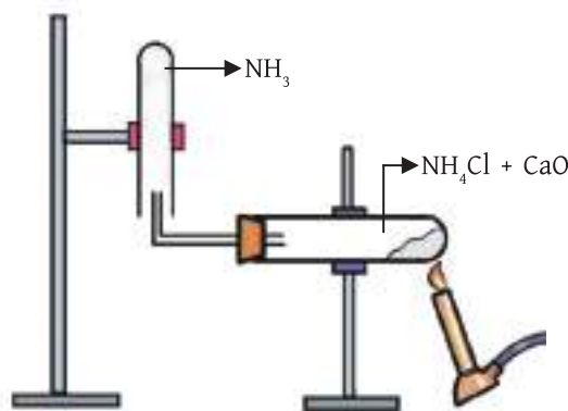
চিত্র ১২.০৪: পরীক্ষাগারে অ্যামোনিয়া গ্যাসের প্রস্তুতি
