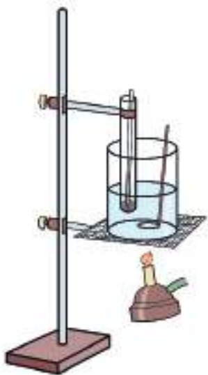
চিত্র ২.০৭: মোমের গলনাঙ্ক নির্ণয়
