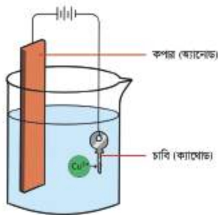
চিত্র ১০.১১: চাবির উপর কপার ধাতুর ইলেকট্রোপ্লেটিং
