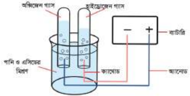
চিত্র ৮.০৬: পানির তড়িৎ বিশ্লেষণ
