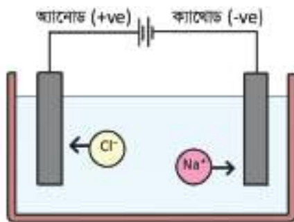
চিত্র ৮.০৪: তড়িৎ বিশ্লেষণ কোষে সোডিয়াম ক্লোরাইডের তড়িৎ বিশ্লেষণ
