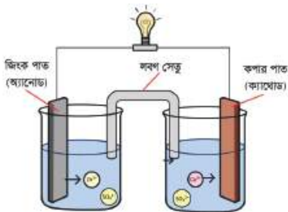
চিত্র ৮.০৮: গ্যালভানিক (ডেনিয়েল) কোষ
