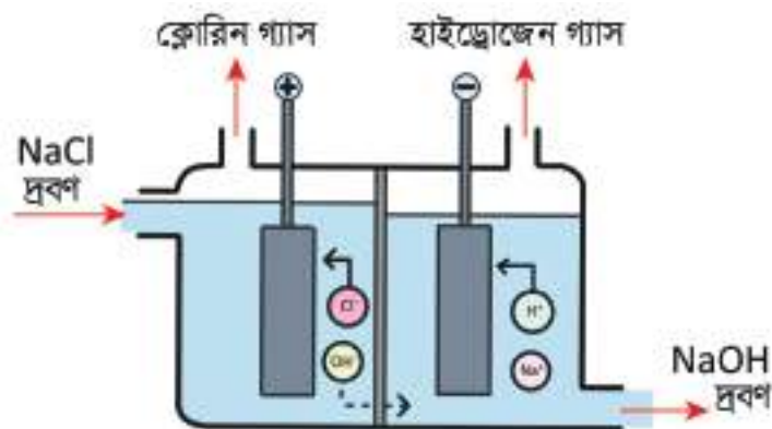
চিত্র ৮.০৫: সোডিয়াম ক্লোরাইড দ্রবণের তড়িৎ বিশ্লেষণ
