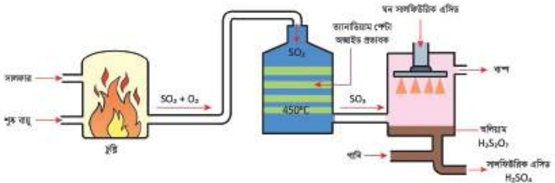
চিত্র ১০.১৩: স্পর্শ পদ্ধতিতে সালফিউরিক এসিড ( H_2SO_4 ) প্রস্তুতি
