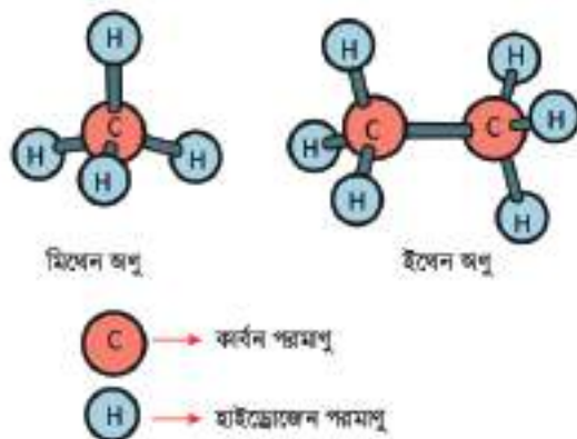
চিত্র ১১.০৩: মিথেন এবং ইথেন
