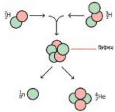
চিত্র ৮.১৪: নিউক্লিয়ার ফিউশন বিক্রিয়া
