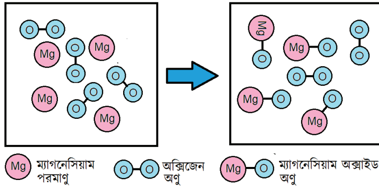
চিত্র ৬.০২: এখানে ম্যাগনেসিয়াম ধাতু লিমিটিং বিক্রিয়ক
