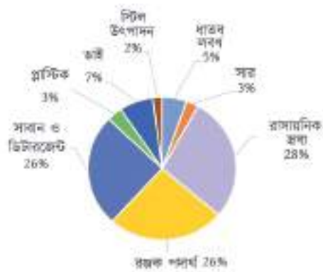
চিত্র ১০.১৪: সালফিউরিক এসিডের ব্যবহার
