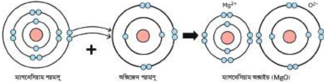
চিত্র ৫.০৭: ম্যাগনেসিয়াম অক্সাইড গঠন
