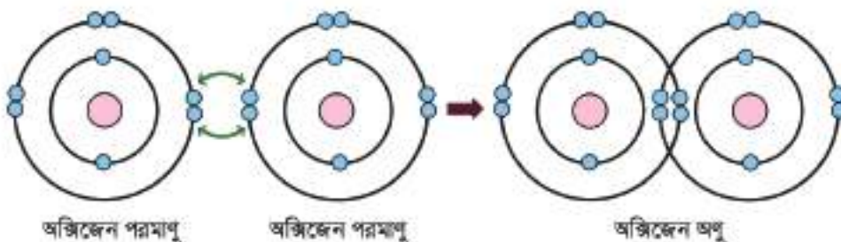
চিত্র ৫.০৯: অক্সিজেন অণুতে সমযোজী বন্ধন গঠন
