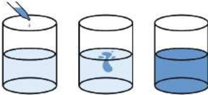
চিত্র ২.০৩: তরল (পানি) মাধ্যমে তরল পদার্থ (নীলের দ্রবণ)
