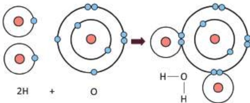
চিত্র ৫.১০: দুটি ( O-H ) সমযোজী বন্ধনের মাধ্যমে পানির অণুতে সমযোজী বন্ধন গঠন
