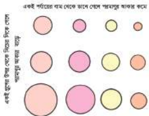
চিত্র ৪.০১: পরমাণুর আকারের পর্যায়বৃত্ত ধর্ম
