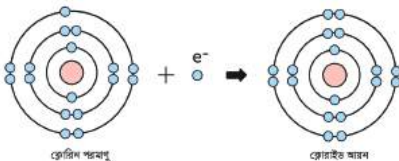
চিত্র ৫.০৫: ঋণাত্মক \text{Cl}^- আয়ন গঠন
