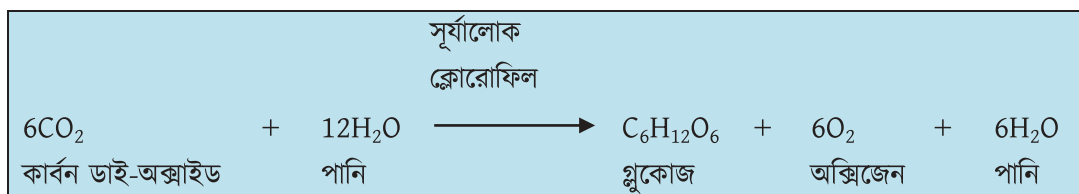
চিত্র ৮.০৩: সালোকসংশ্লেষণ প্রক্রিয়া
