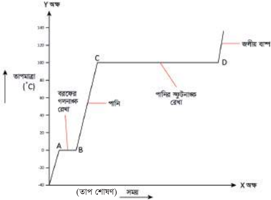
চিত্র ২.০৯: বরফে তাপ প্রদানের লেখচিত্র
