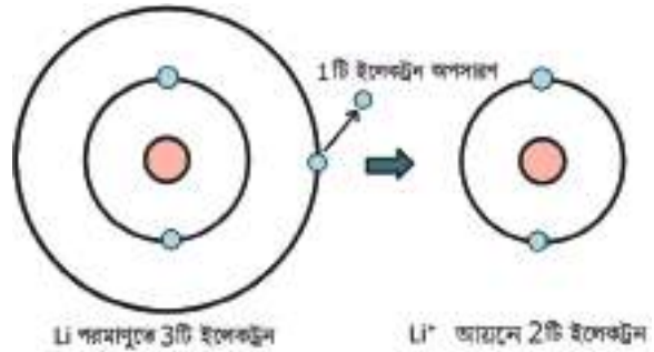
চিত্র ৪.০২: মৌলের আয়নিকরণ
