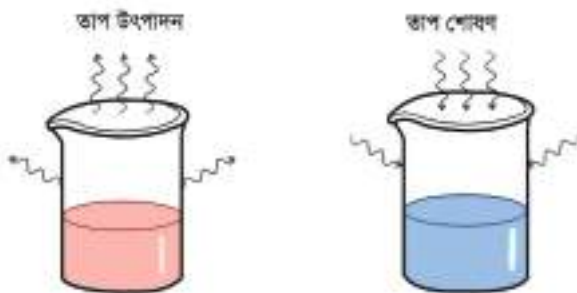
চিত্র ৮.০১: তাপ উৎপাদন ও তাপ শোষণ
