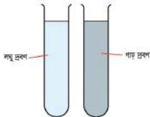
চিত্র ৬.০১: লঘু দ্রবণ এবং গাঢ় দ্রবণ
