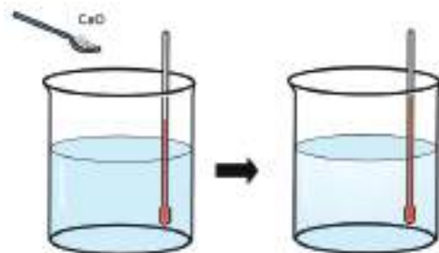
চিত্র ৮.১৮: বিকারে পানি ও চুনের দ্রবণ
