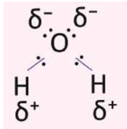
চিত্র ৫.১১: \delta^+ ও \delta^- দিয়ে আংশিক ধনাত্মক আধান এবং আংশিক ঋণাত্মক আধানকে বোঝানো হচ্ছে
