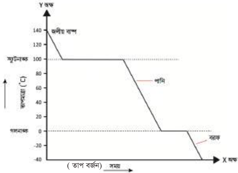
চিত্র ২.১০: জলীয় বাষ্পকে শীতলকরণের লেখচিত্র
