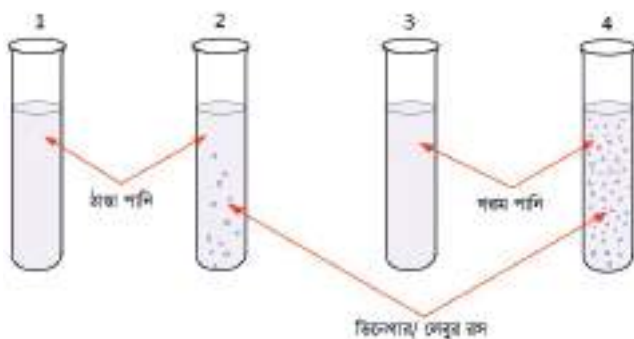
চিত্র ৭.০৪: সোডিয়াম কার্বনেট দ্রবণের সাথে ভিনেগার বা এসিটিক এসিডের বিক্রিয়া
