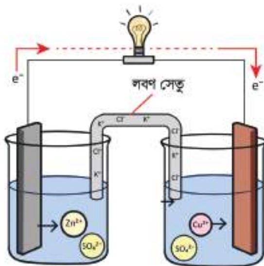
চিত্র ৮.০৯: কোষে ব্যবহৃত লবণ সেতু
