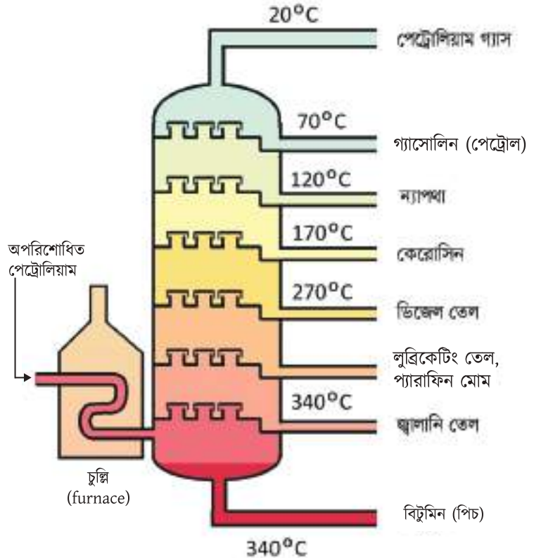
চিত্র ১১.০১: পেট্রোলিয়ামের আংশিক পাতন
