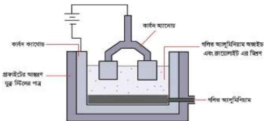
চিত্র ১০.০৭: তড়িৎ বিশ্লেষণের পদ্ধতিতে অ্যালুমিনিয়াম ধাতু নিষ্কাশন
