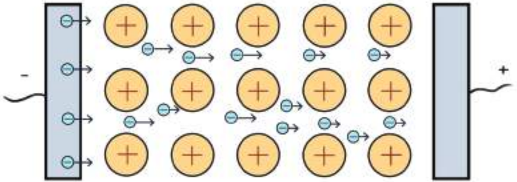
চিত্র ৫.১৫: ধাতুর বিদ্যুৎ পরিবহনের কৌশল
