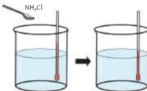
চিত্র ৮.১৭: বিকারে \text{NH}_4\text{Cl} এর দ্রবণ
