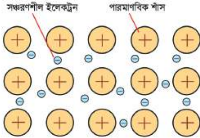
চিত্র ৫.১৪: ধাতব বন্ধন
