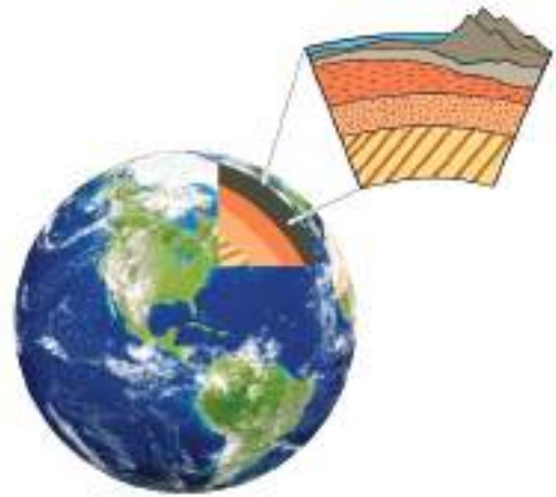
চিত্র ১০.০৩: শিলার বিভিন্ন স্তর
