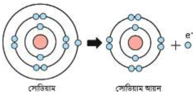
চিত্র ৫.০৪: সোডিয়াম ক্যাটায়ন ( \text{Na}^+ ) গঠন
