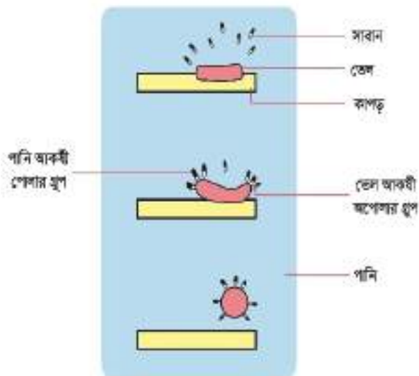
চিত্র ১২.০২: সাবান কিংবা ডিটারজেন্ট দিয়ে ময়লা পরিষ্কার করার কৌশল
