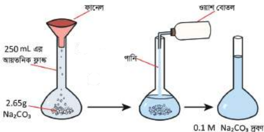
চিত্র ৬.০৩: ০.১ মোলার সোডিয়াম কার্বনেট দ্রবণ প্রস্তুতি
