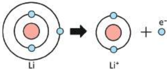
চিত্র ৫.০৩: লিথিয়াম ক্যাটায়ন ( \text{Li}^+ ) গঠন
