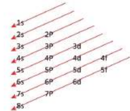
চিত্র ৩.০৪: অরবিটালের শক্তিক্রম
