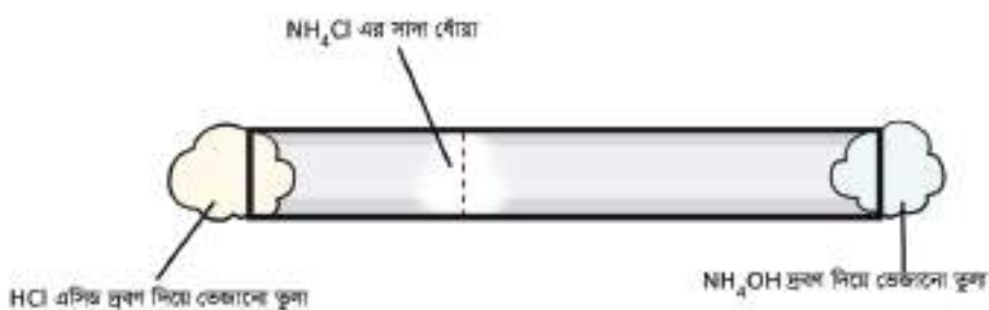
চিত্র ২.০৪: দুটি গ্যাসের ব্যাপন
