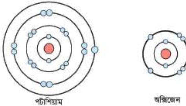
চিত্র ৫.০১: (a) পটাশিয়ামের যোজ্যতা ইলেকট্রন (b) অক্সিজেনের যোজ্যতা ইলেকট্রন
