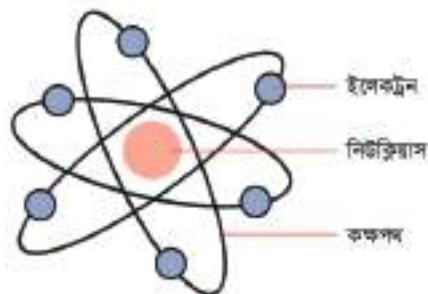
চিত্র ৩.০১: রাদারফোর্ডের পরমাণু মডেল
