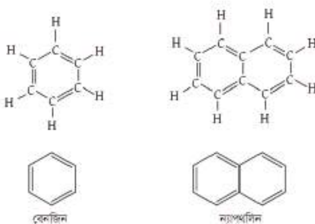
চিত্র ১১.০২: অ্যারোমেটিক যৌগ বেনজিন ( C_6H_6 ), এবং ন্যাপথলিন ( C_{10}H_8 )
