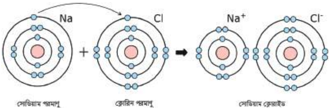
চিত্র ৫.০৬: সোডিয়াম ক্লোরাইড গঠন
