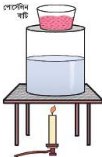
চিত্র ১২.০৩: সাবান প্রস্তুতি
