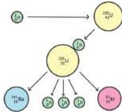
চিত্র ৮.১৩: নিউক্লিয়ার ফিশন বিক্রিয়া
