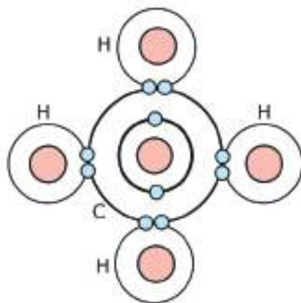
চিত্র ৫.০২: মিথেন অণুতে অষ্টক নিয়ম
