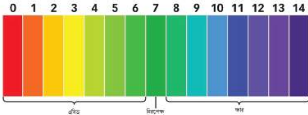
চিত্র ৯.০১: pH স্কেল (ইউনিভার্সাল ইন্ডিকেটরের বিভিন্ন pH এ বর্ণ)
