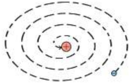
চিত্র ৩.০২: ইলেকট্রন শক্তি হারিয়ে নিউক্লিয়াসে পতিত হচ্ছে
