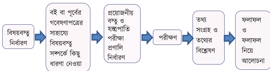
চিত্র ১.০২: রসায়নে অনুসন্ধান বা গবেষণা প্রক্রিয়ার বিভিন্ন ধাপ
