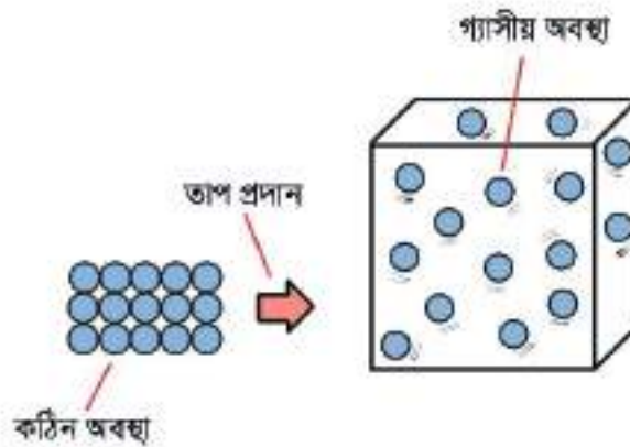
চিত্র ২.১১: উদ্বায়ী পদার্থের উর্ধ্বপাতন
