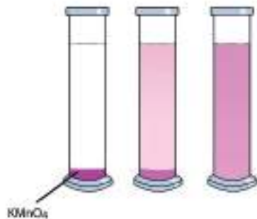
চিত্র ২.০২: পানিতে \text{KMnO}_4 এর ব্যাপন
