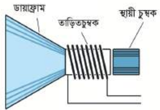
চিত্র ১২.০৮: স্পিকারে তাড়িতচুম্বক ব্যবহার করা হয়।
