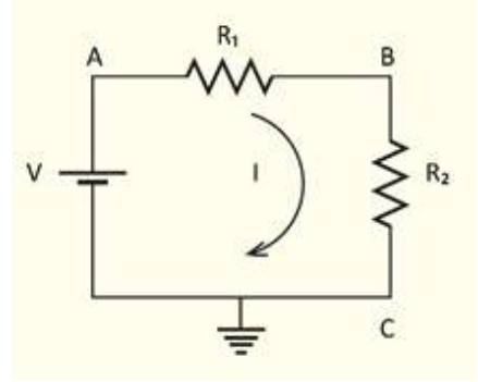
চিত্র ১১.১১: একটি বর্তনী বা সার্কিটে দুটি রোধ পরপর লাগানো।
