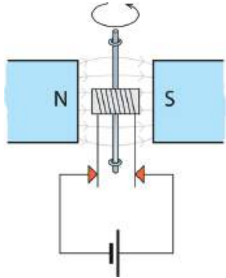
চিত্র ১২.১১: একটি বৈদ্যুতিক মোটর।
