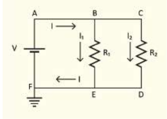
চিত্র ১১.১৩: একটি সার্কিটে দুটি রোধ সমান্তরালভাবে রাখা।
