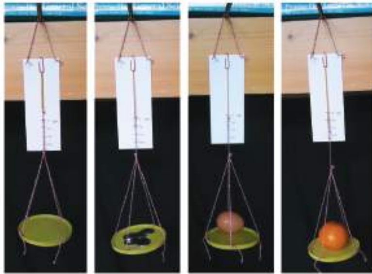
চিত্র ৩.১১: রাবার ব্যান্ড দিয়ে তৈরি স্প্রিং ব্যালেন্স।
