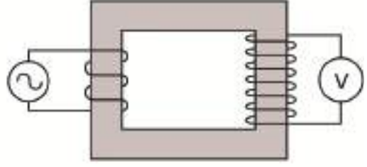
চিত্র ১২.১৩: ট্রান্সফর্মারের প্রাইমারি কয়েলে এসি বিভব পার্থক্য প্রয়োগ করা হলে সেকেন্ডারি কয়েলে সেটি বিভব পার্থক্য তৈরি করে।
