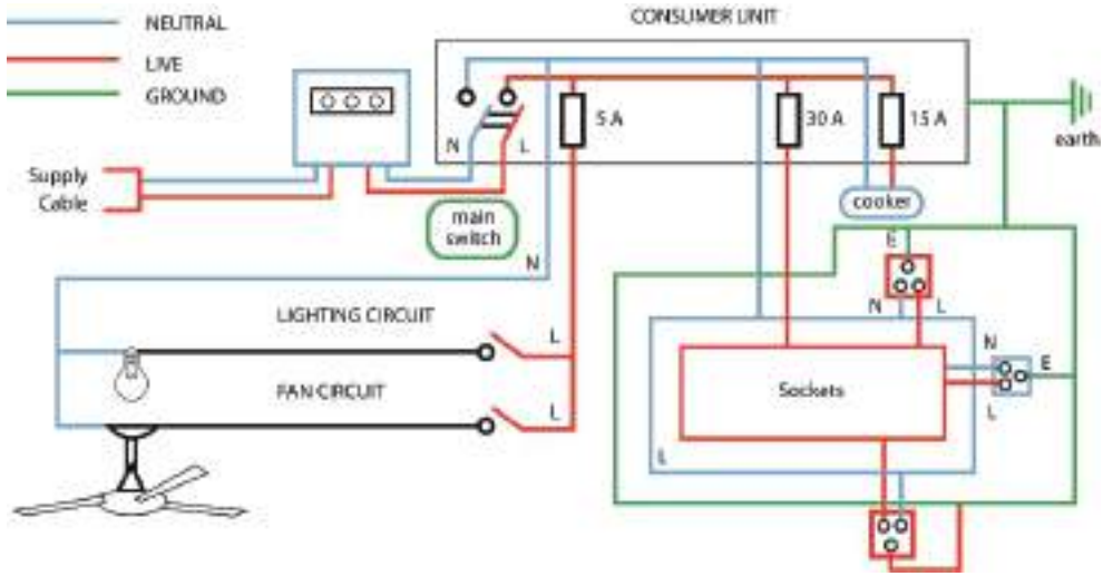
চিত্র ১১.১৭: একটি বাসায় বিদ্যুৎ সরবরাহ করার জন্য সম্ভাব্য বিদ্যুৎ বর্তনী।
