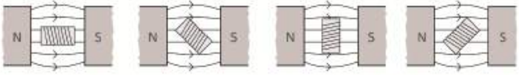
চিত্র ১২.১০: বৈদ্যুতিক মোটর একটি তাড়িতচুম্বকের ভেতর দিয়ে এমনভাবে পরিবর্তী বিদ্যুৎ প্রবাহ করানো হয়, যেন সব সময়েই এটি ঘুরতে থাকে।
