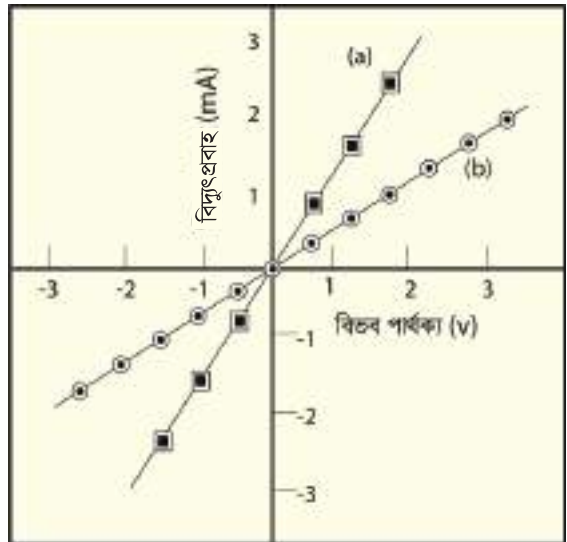
চিত্র ১১.০৪ : রেজিস্ট্যান্সের কারণে বিভব পার্থক্যের সাপেক্ষে বিদ্যুৎপ্রবাহ।
