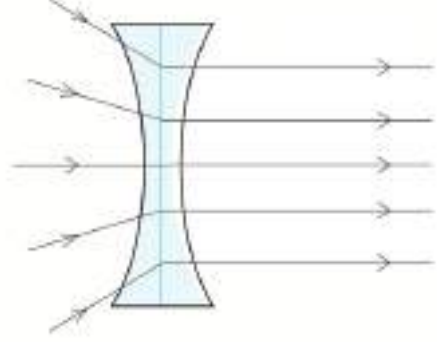
চিত্র ৯.১৯: অবতল লেন্সের ভেতর দিয়ে যাবার সময় অভিসারী রশ্মি সমান্তরাল হয়ে যাবে।
