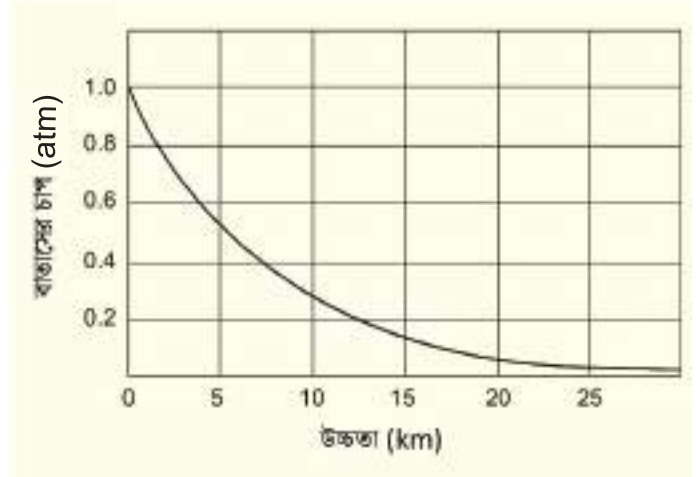
চিত্র ৫.০৯: উচ্চতার সাথে বাতাসের চাপ কমে যায়
