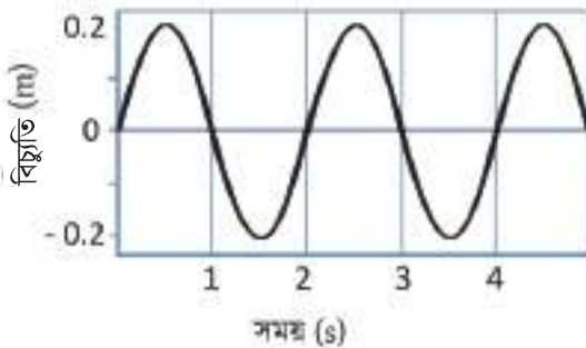
চিত্র ৭.০৭: সময়ের সাপেক্ষে একটি তরঙ্গ।
