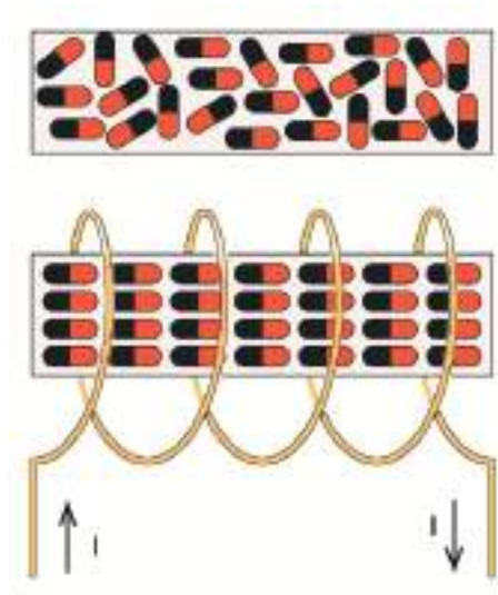
চিত্র ১২.০৭: বিদ্যুৎ প্রবাহের কারণে এলোমেলোভাবে থাকা ছোট ছোট চুম্বক সারিবদ্ধ হয়ে শক্তিশালী চৌম্বক ক্ষেত্র তৈরি করে।
