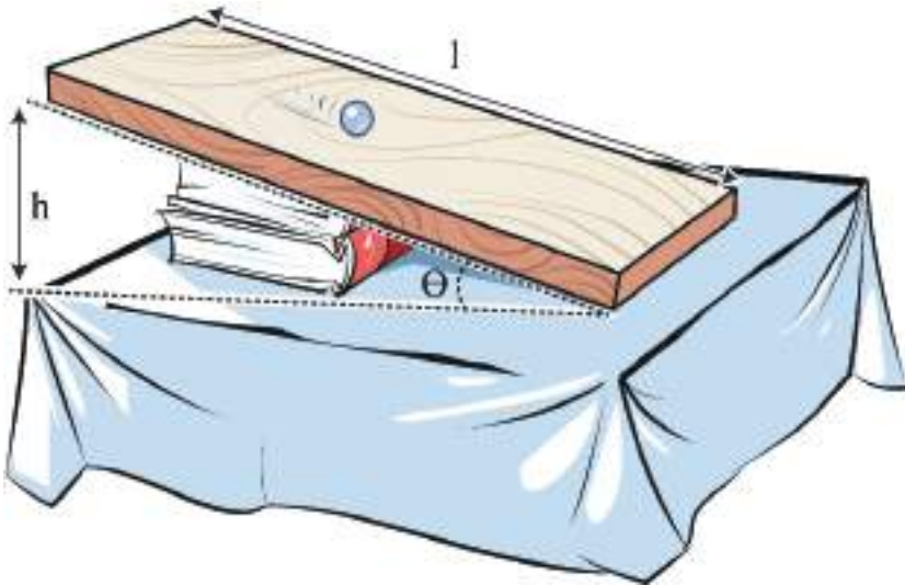
চিত্র ২.১০: ঢালু পথে একটি মারবেল গড়িয়ে দেওয়া হয়েছে।
