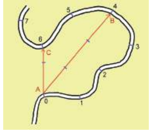
চিত্র ২.০৪ : A বিন্দু থেকে শুরু করে আঁকাবাঁকা পথে সাইকেল চালিয়ে যাওয়া।
