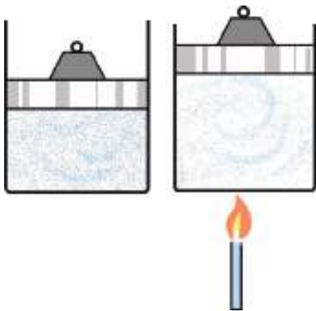
চিত্র ৬.০৭: তাপ প্রয়োগ করলে বাতাসের আয়তন বেড়ে যায়।
