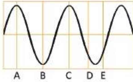
চিত্র ৭.০৯ : ভিন্ন ভিন্ন অবস্থানে একটি তরঙ্গের দশা
