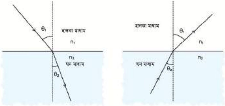
চিত্র ৯.০২: হালকা মাধ্যম থেকে ঘন মাধ্যমে হওয়ার সময় আলো লম্বের দিকে বেঁকে যায়। ঘন মাধ্যম থেকে হালকা মাধ্যমে যাবার সময় আলো লম্ব থেকে দূরে সরে যায়।
