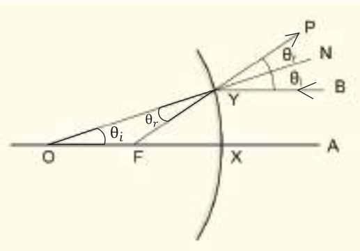
চিত্র ৮.১৮: একটি গোলায় উত্তল আয়না আসলে একটা গোলকের অংশ।
