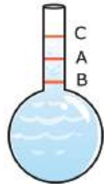
চিত্র ৬.০৬: সত্যিকার এবং আপাত প্রসারণ।
