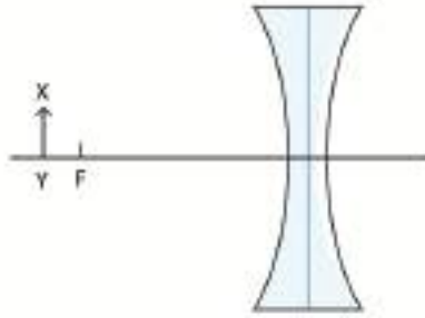
চিত্র ৯.২৮: অবতল লেন্সের ফোকাস দূরত্বের বাইরে রাখা একটি বস্তু।
