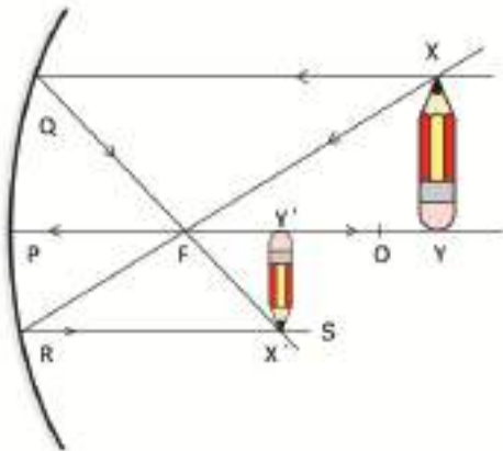
চিত্র ৮.২৪: অবতল আয়নায় একটি বস্তু ফোকাস দূরত্বের দ্বিগুণ দূরত্বের বাইরে রাখলে প্রতিবিম্বটি উল্টো এবং ছোট হয়।
