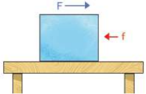
চিত্র ৩.১৫: একটি ভরের উপর বল প্রয়োগ করলে ঘর্ষণের জন্যে বিপরীত দিকে একটি বল তৈরি হতে পারে।
