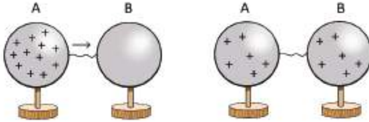
চিত্র ১১.০১ : চার্জ সংযুক্ত গোলক থেকে চার্জহীন গোলকে বিদ্যুৎ প্রবাহ।
