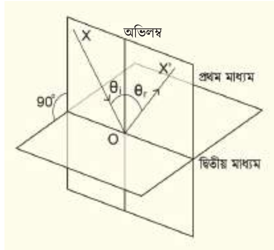
চিত্র ৮.০৩: প্রথম মাধ্যম থেকে দ্বিতীয় মাধ্যমে আলোর প্রতিফলন।
