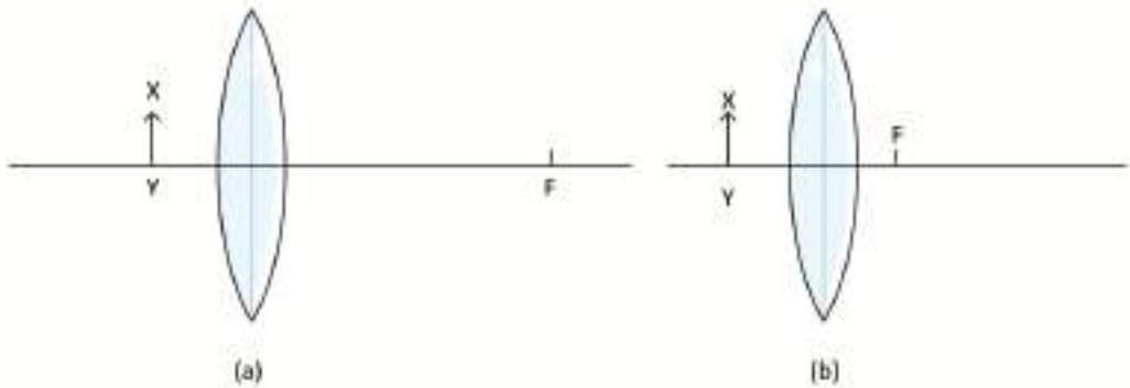
চিত্র ৯.২৯: (a) উত্তল লেন্সের ফোকাস দূরত্বের ভেতরে রাখা একটি বস্তু (b) উত্তল লেন্সের ফোকাস দূরত্বের বাইরে রাখা একটি বস্তু।
