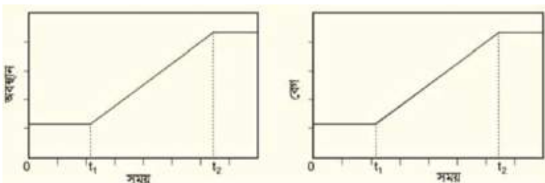
চিত্র ৩.০১: অবস্থান-সময় ও বেগ-সময়ের দুটি লেখচিত্র।
