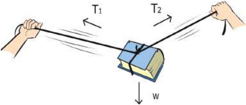
চিত্র ৩.০৩: দুই পাশ থেকে তুমি যত জোরেই টানার চেষ্টা করো না কেন, তুমি কখনোই দড়িটা পুরোপুরি সোজা করতে পারবে না, কারণ তাহলে বইয়ের ওজনের বলটিকে নিষ্ক্রিয় করা যাবে না।
