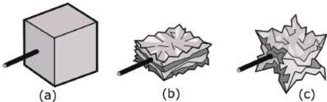
চিত্র ৫.০৭: (a) তে দেখানো কিউবটির ভেতর থেকে পাম্প করে বাতাস সরিয়ে নিলে যদি শুধু উপর থেকে চাপ দিত তাহলে (b) ছবির মতো চ্যাপ্টা হয়ে যেত। কিন্তু যেহেতু চারদিক থেকে চাপ আসে তাই (c) ছবির মতো সংকুচিত হয়।
