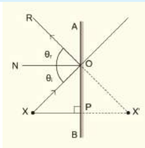
চিত্র ৮.০৯: X অবস্থানের বস্তুটির প্রতিবিম্ব দেখার জন্য XP এবং XO এই দুটি আলোক রশ্মি ব্যবহার করাই যথেষ্ট।
