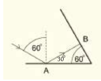
চিত্র ৮.১৩: 60^\circ কোণে রাখা দুটি আয়নার একটিতে 60^\circ কোণে আপতিত আলো।
