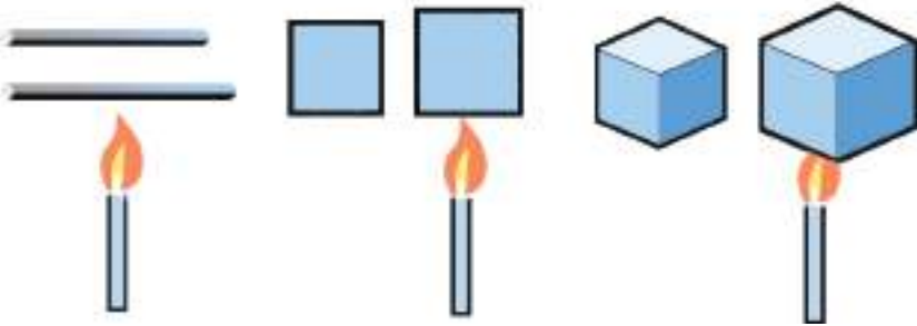
চিত্র ৬.০৪: তাপ প্রয়োগ করলে কঠিন পদার্থের দৈর্ঘ্য, প্রস্থচ্ছেদ এবং আয়তন বেড়ে যায়।
