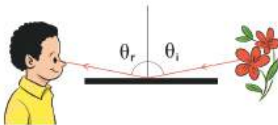
চিত্র চ.০৫: আপাতন কোণ বেশি হলে প্রতিফলন অনেক বেশি হয়।
