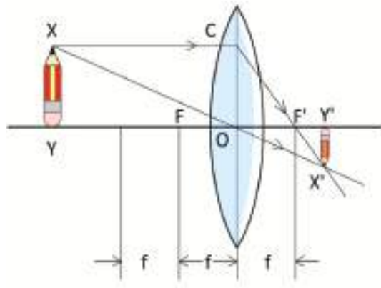
চিত্র ৯.২৬: দ্বিগুণ ফোকাস দূরত্বের বাইরে বস্তু রাখা হলে তার ছোট, উল্টো ও বাস্তব প্রতিবিম্ব তৈরি হয়।
