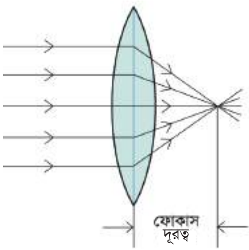
চিত্র ৯.২১: উত্তল লেন্সের ভেতর দিয়ে যাবার সময় সমান্তরাল রশ্মি ফোকাস বিন্দুতে কেন্দ্রীভূত হয়।
