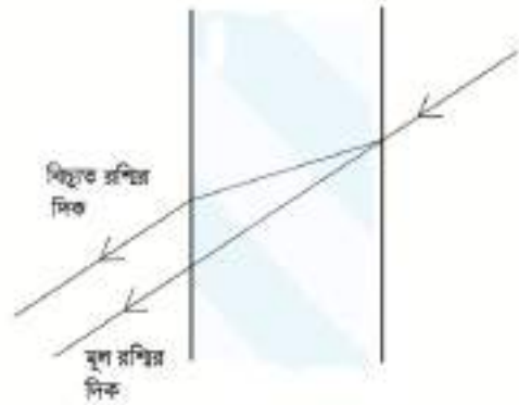
চিত্র ৯.১৬: পুরু কাচের ভেতর দিয়ে যাবার সময় প্রতিসরণের কারণে মূল রশ্মি থেকে আলোক রশ্মি বিচ্যুত হয়।
