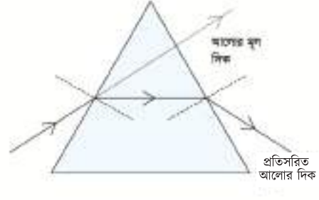
চিত্র ৯.১২: প্রিজমের আলোক রশ্মির দিক প্রিজমের ভূমির দিকে বেঁকে যায়।
