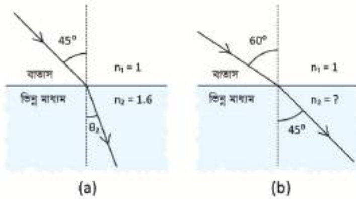
চিত্র ৯.০৮: (a) আলো 45^\circ কোণে আপতিত হচ্ছে (b) আলো 60^\circ কোণে আপতিত হয়ে 45^\circ কোণে প্রতিসরিত হচ্ছে।
