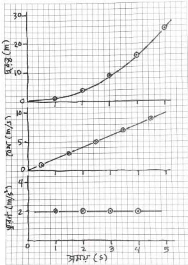
চিত্র ২.০৯: দূরত্ব-সময় থেকে বেগ-সময় এবং বেগ-সময় থেকে ত্বরণ-সময় বের করে একটি গ্রাফ পেপারে লেখচিত্র আঁকা হয়েছে।
