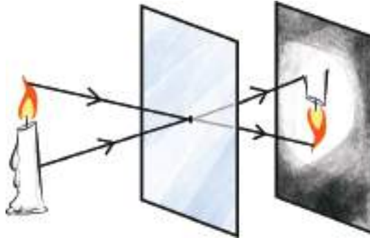
চিত্র ৮.১৪: সূক্ষ্ম ফুটো দিয়ে কোনো বস্তুর প্রতিবিম্ব তৈরি করা সম্ভব।
