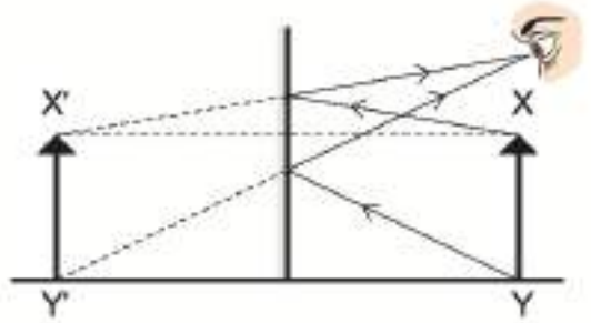
চিত্র ৮.১০: XY বস্তুটির প্রতিবিম্ব X'Y'
