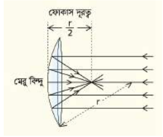
চিত্র ৮.২১: অবতল আয়নার ফোকাস দূরত্ব গোলকের ব্যাসার্ধের অর্ধেক।
