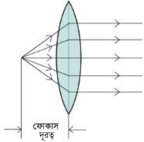
চিত্র ৯.২২: ফোকাস দূরত্বে আলোক বিন্দু রাখা হলে উত্তল লেন্স সেটিকে সমান্তরাল রশ্মিতে পরিণত করে।
