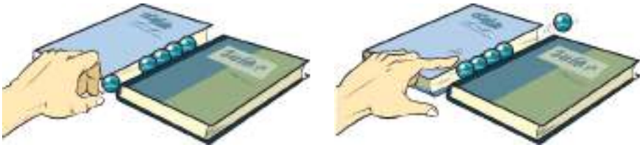
চিত্র ৩.০৫ : ভরবেগ এবং শক্তির সংরক্ষণশীলতার পরীক্ষা
