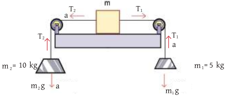
চিত্র ৩.১০: কপিকল দিয়ে একটি ভরকে দুই পাশে থেকে দুটি ওজনের মাধ্যমে বল প্রয়োগ করা হচ্ছে
