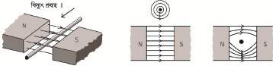
চিত্র ১২.০৯: চৌম্বক ক্ষেত্রে বিদ্যুৎপ্রবাহী তার রাখা হলে সেটি বল অনুভব করে।
