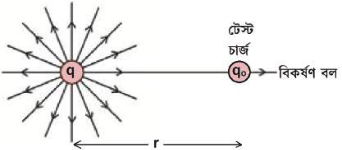
চিত্র ১০.১৪: একটি ধনাত্মক আধান q থেকে r দূরত্বে একটি ক্ষুদ্র টেস্ট চার্জ q_0 কে আনা হলো
