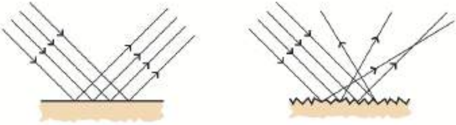
চিত্র ৮.০৭: মসৃণ পৃষ্ঠে আলো প্রতিফলিত হয় কিন্তু অমসৃণ পৃষ্ঠে আলো বিচ্ছুরিত হয়।
