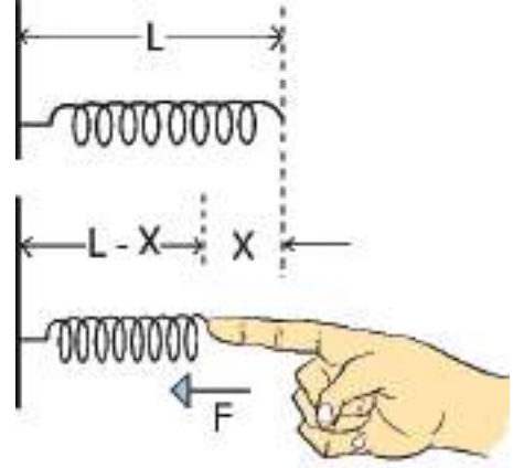
চিত্র ৪.০২: স্প্রিংয়ের স্থিরাবস্থা এবং বল প্রয়োগ করে সংকুচিত অবস্থা
