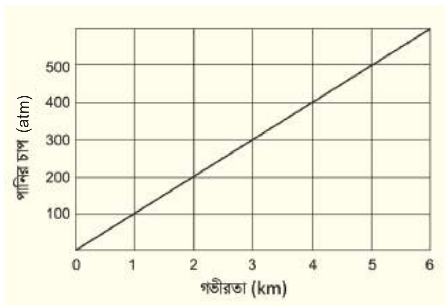
চিত্র ৫.০৩: পানির গভীরতার সাথে সাথে পানির চাপ বেড়ে যায়।
