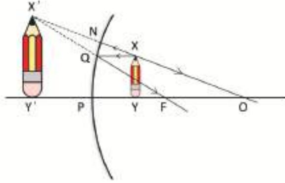
চিত্র ৮.২২: অবতল আয়নায় একটি বস্তু ফোকাস দূরত্বের ভেতরে রাখা হলে প্রতিবিম্বটি বড় দেখায়।
