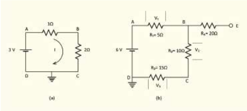
চিত্র ১১.০৯: ব্যাটারি এবং একাধিক রেজিস্টর বা রোধ দিয়ে তৈরি দুটি সার্কিট।
