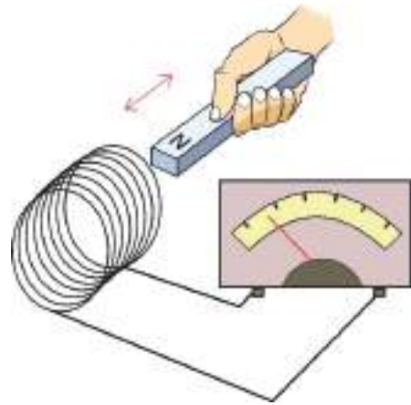
চিত্র ১২.১২: সলিনয়েডে চুম্বক প্রবেশ করানোর সময় বিদ্যুৎপ্রবাহ দেখা যায়।
