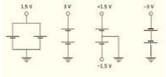
চিত্র ১১.০৩: দুটি ব্যাটারি সেল দিয়ে বিভিন্ন পজিটিভ বা নেগেটিভ ভোল্টেজ তৈরি করা।
