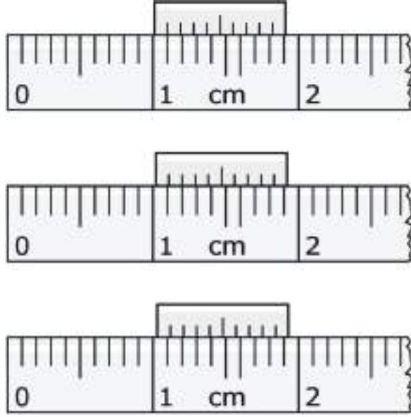
চিত্র ১.০৭: এক, দুই এবং তিন ঘর সরে যাওয়া ভার্নিয়ার স্কেল।
