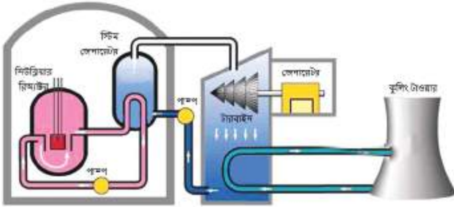
চিত্র ৪.০৫: নিউক্লিয়ার শক্তি কেন্দ্রের গঠন।
