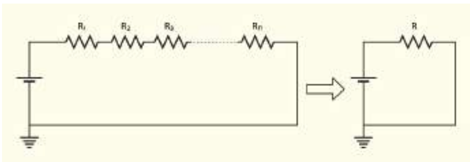
চিত্র ১১.১২: অনেকগুলো পর্যায়ক্রম রোধ বা রেজিস্টরকে একটি তুল্য রোধ বা রেজিস্টর হিসেবে কল্পনা করা যায়।
