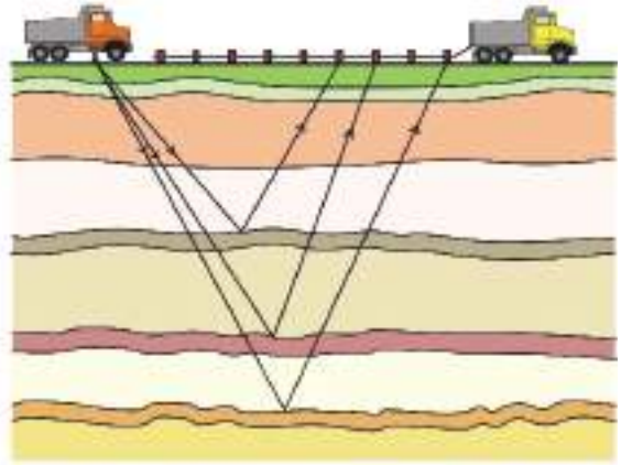
চিত্র ৭.১৩: শব্দ তরঙ্গে প্রতিফলন থেকে ভূপৃষ্ঠের ভিন্ন ভিন্ন স্তর সম্পর্কে তথ্য জানা যায়।
