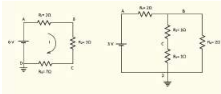
চিত্র ১১.১৮: (a) এবং (b) ব্যাটারি ও রোধ সংযুক্ত দুটি সার্কিট।
