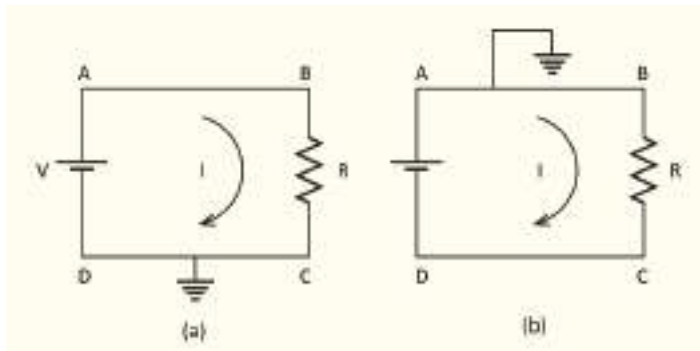
চিত্র ১১.০৮: একটি ব্যাটারি এবং একটি রোধ বা রেজিস্টর সংযুক্ত দুটি বর্তনী বা সার্কিট।
