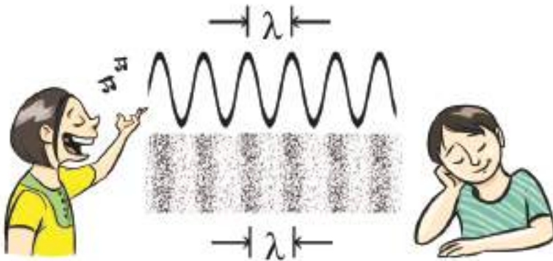
চিত্র ৭.০৪: শব্দ হচ্ছে বাতাসের চাপের কারণে সংকোচন এবং প্রসারণের একটি অনুদৈর্ঘ্য তরঙ্গ। এখানে \lambda হচ্ছে তরঙ্গদৈর্ঘ্য।
