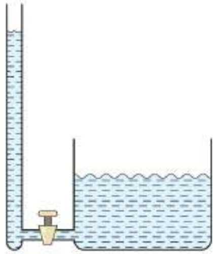
চিত্র ৬.০১: তাপমাত্রা তরলের উচ্চতার মতো, তাপ তরলের আয়তনের মতো।
