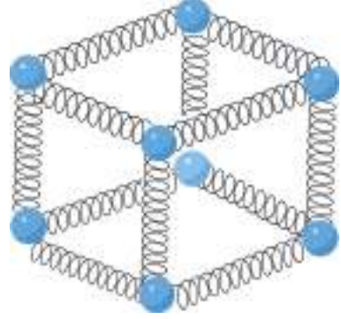
চিত্র ৬.০৩: অণুগুলো একটি অন্যটির সাথে স্প্রিং দিয়ে যুক্ত কল্পনা করে নেওয়া যায়।
