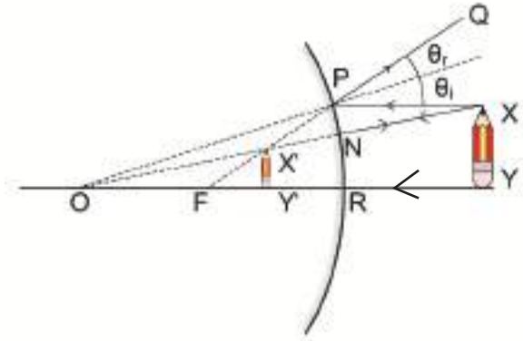
চিত্র ৮.১৯: উত্তল আয়নায় একটি বস্তু XY ফোকাস দূরত্বের ভেতরে রাখা হলে প্রতিবিম্ব X'Y' ছোট দেখায়।
