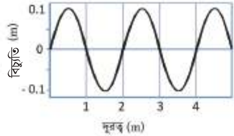
চিত্র ৭.০৬: অবস্থানের সাপেক্ষে একটি তরঙ্গ।
