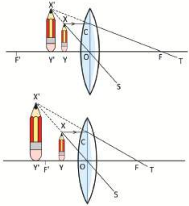
চিত্র ৯.২৭: যে লেন্সের ফোকাস দূরত্ব যত কম সেই লেন্সে জিনিসটিকে তত বড় দেখায়।
