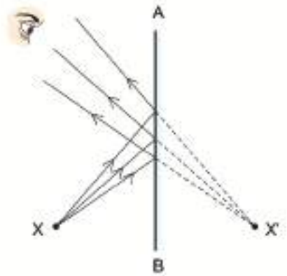
চিত্র ৮.০৮: X বস্তুটির প্রতিবিম্ব X' অবস্থানে দেখা যাবে।
