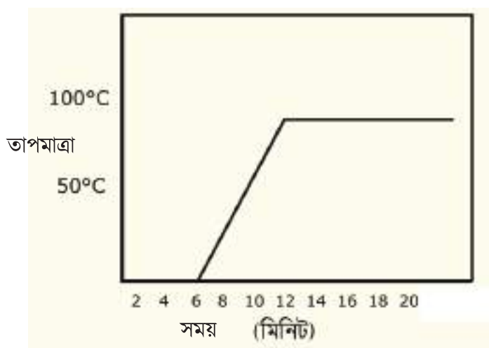
চিত্র ৬.১০: বরফ গলনের লেখচিত্র
