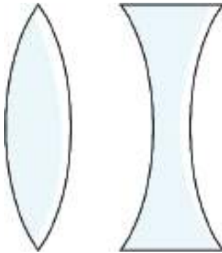
চিত্র ৯.১৪: একটি উত্তল ও একটি অবতল লেন্সের প্রস্থচ্ছেদ
