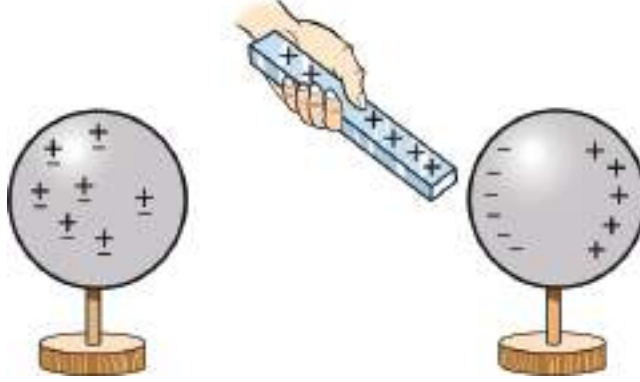
চিত্র ১০.০৪: চার্জবিহীন বস্তুর কাছে চার্জসহ বস্তু আনা হলে বিপরীত চার্জ আবেশিত হয়।
