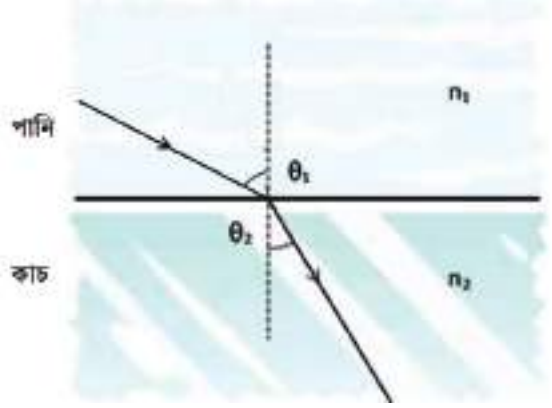
চিত্র ৯.০৫: পানি ও কাচের ভেতর আলোর প্রতিসরণ।
