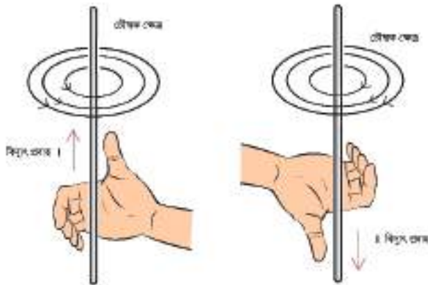
চিত্র ১২.০৩: বিদ্যুৎপ্রবাহকে ঘিরে তৈরি চৌম্বক ক্ষেত্রের দিক নির্ণয়ের ডানহাতি নিয়ম।
