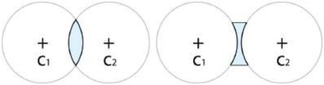
চিত্র ৯.১৫: উত্তল এবং অবতল লেন্সকে দুটি গোলকের অংশ হিসেবে কল্পনা করা যায়
