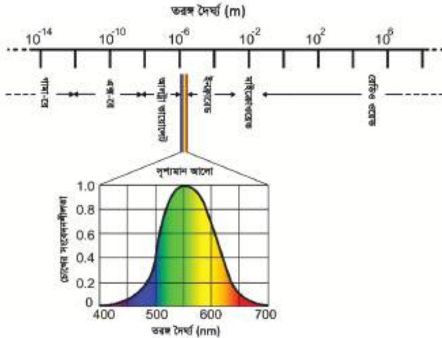
চিত্র ৮.০১ : আলোর স্পেকট্রাম এবং ভিন্ন ভিন্ন রংয়ে চোখের সংবেদনশীলতা।
