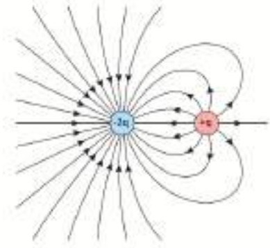
চিত্র ১০.১৩: চার্জ এবং দ্বিগুণ পরিমাণ বিপরীত চার্জের জন্য বলরেখা।
