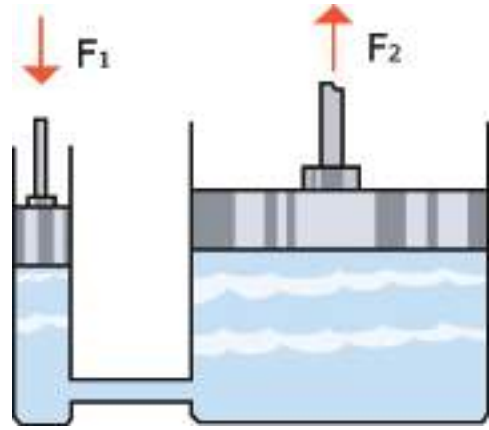
চিত্র ৫.০৫: F_1 বল প্রয়োগ করলে প্রস্থচ্ছেদের উপর নির্ভর করে অন্য দিকে F_2 বল পাওয়া যায়।
