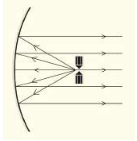
চিত্র ৮.২৭: ফোকাস দূরত্বে তীব্র আলো তৈরি করলে সেটি অবতল আয়নায় প্রতিফলিত হয়ে সমান্তরাল আলো হিসেবে বের হয়ে আসবে।
