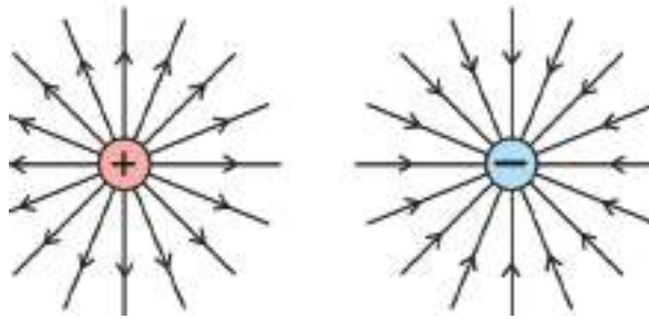
চিত্র ১০.১১: পজিটিভ চার্জ থেকে বলরেখা চারদিকে ছড়িয়ে পড়ে এবং নেগেটিভ চার্জের দিকে বলরেখা কেন্দ্রীভূত হয়।
