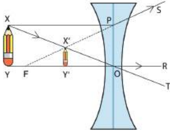
চিত্র ৯.২০: অবতল লেন্সে একটি বস্তুকে ছোট দেখায়।
