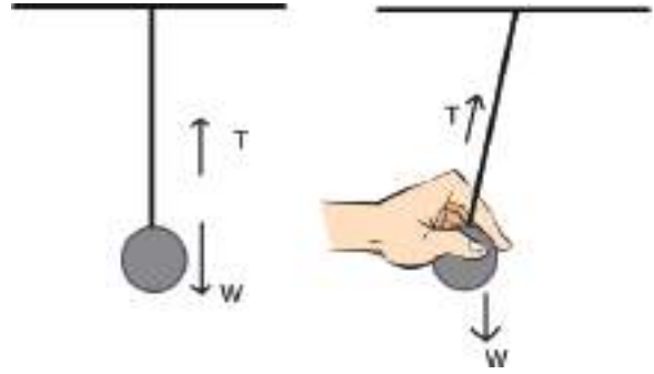
চিত্র ৩.০২: প্রথম ছবিতে বলের একটি সাম্যাবস্থা আছে।
