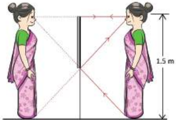
চিত্র ৮.১২: পূর্ণদৈর্ঘ্য প্রতিবিম্ব দেখার জন্য পূর্ণদৈর্ঘ্য আয়নার প্রয়োজন হয় না।
