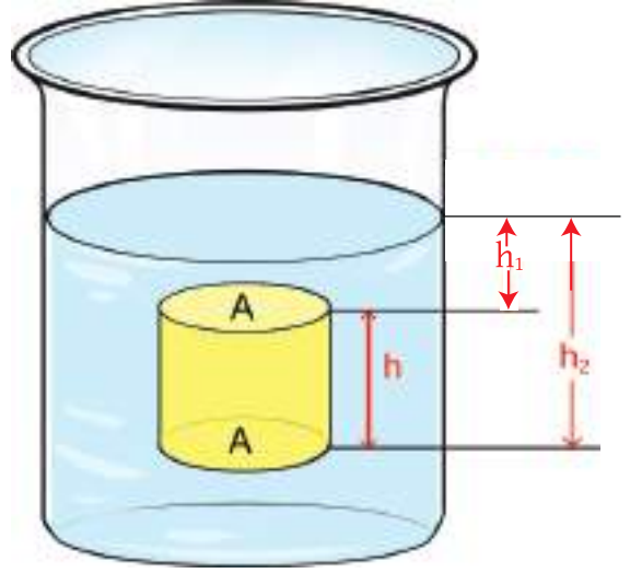
চিত্র ৫.০৪: একটি বস্তু যতটুকু তরল অপসারিত করে তার সমপরিমাণ ওজন হারায়।
