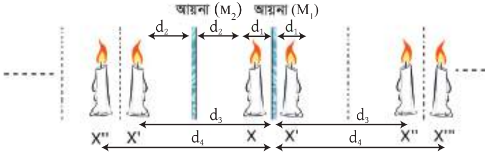
চিত্র চ.০৪: দুটি সমান্তরাল আয়নার মাঝখানে একটি মোমবাতি X রাখা হলে তার প্রতিবিম্ব X' এবং X' প্রতিবিস্মের প্রতিবিম্ব X'' , X''' ... তৈরি হতে থাকে।
