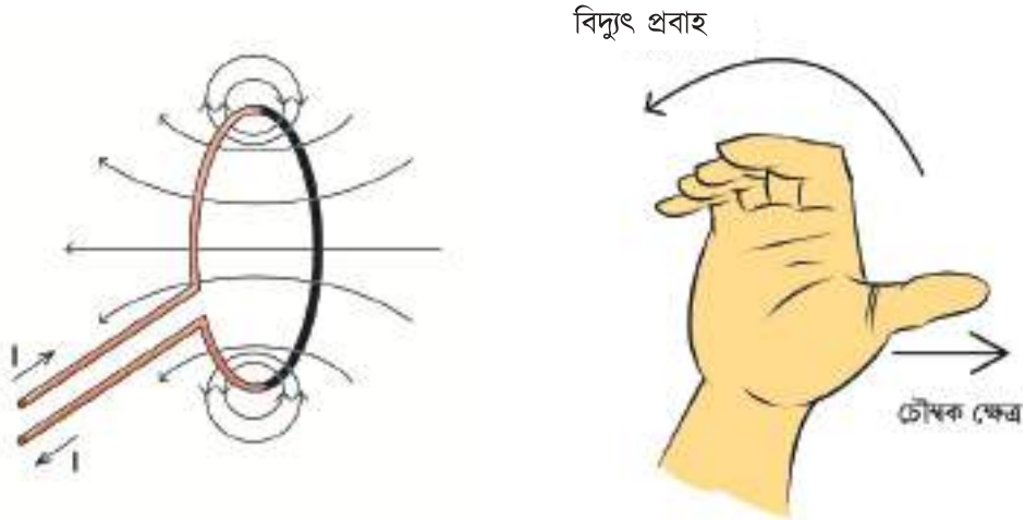
চিত্র ১২.০৫: লুপের ভেতর দিয়ে বিদ্যুৎপ্রবাহের কারণে তৈরি চৌম্বক ক্ষেত্র।
