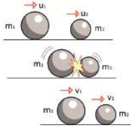
চিত্র ৩.০৪: m_1 এবং m_2 পরস্পরকে আঘাত করার পর তাদের বেগ পরিবর্তিত হয়ে v_1 এবং v_2 হয়েছে।
