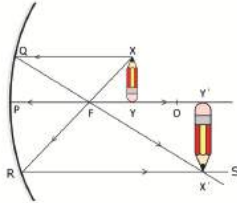
চিত্র ৮.২৩: অবতল আয়নায় একটি বস্তু ফোকাস দূরত্বের বাইরে রাখলে প্রতিবিম্বটি হয় উল্টো।
