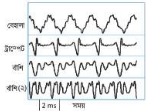
চিত্র ৭.১৪: ভিন্ন ভিন্ন বাদ্যযন্ত্রের শব্দ তরঙ্গ।
