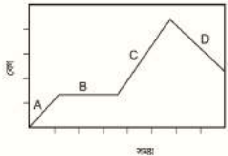
চিত্র ২.০৬: সময়ের সাথে বেগের পরিবর্তন।
