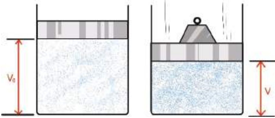
চিত্র ৫.১২: আবদ্ধ বাতাসে চাপ প্রয়োগ করলে বাতাস সংকুচিত হয়।
