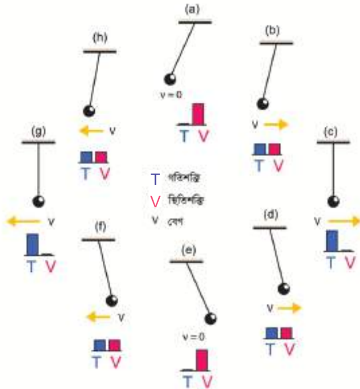
চিত্র ৪.০৪: একটি পেডুলাম দুলছে, গতিশক্তি এবং বিভবশক্তি বাড়লে কমলেও মোট শক্তির পরিমাণ নির্দিষ্ট থাকে।
