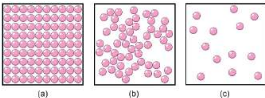
চিত্র ৫.১৩: (a) কঠিন, (b) তরল এবং (c) গ্যাস।
