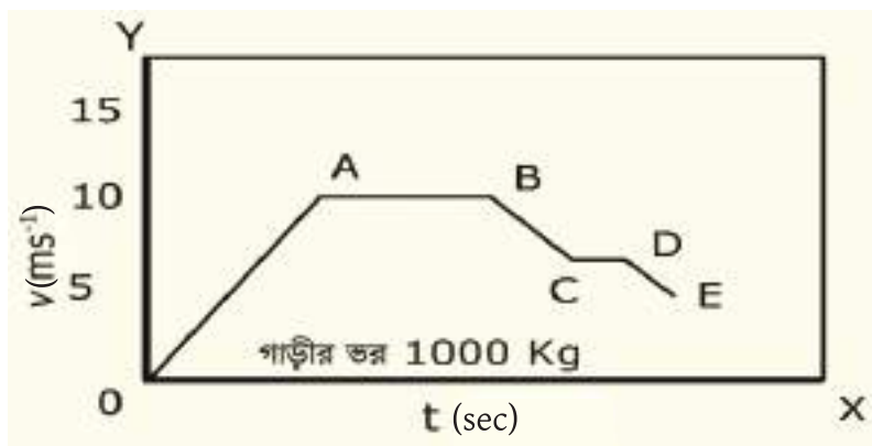
চিত্র ৪.০৭: বেগ-সময় লেখচিত্র
