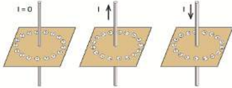
চিত্র ১২.০২: বিদ্যুৎ প্রবাহকে ঘিরে কম্পাসের দিক।
