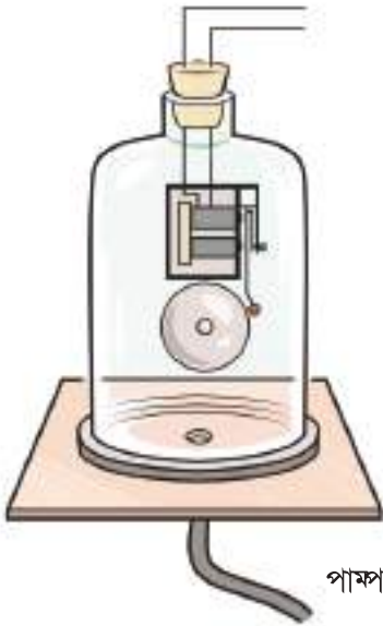
চিত্র ৭.১১: বেলজার থেকে বাতাস পাম্প করে সরিয়ে নিলে কলিং বেলে শব্দটি আর শোনা যাবে না।
