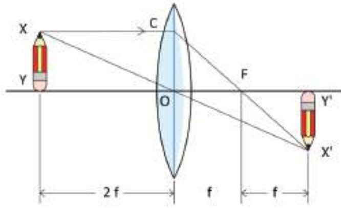
চিত্র ৯.২৫: ঠিক ফোকাস দূরত্বের দ্বিগুণ দূরত্বে কোনো বস্তু রাখা হলে তার প্রতিবিম্বটি হবে বস্তুটির সমান।
