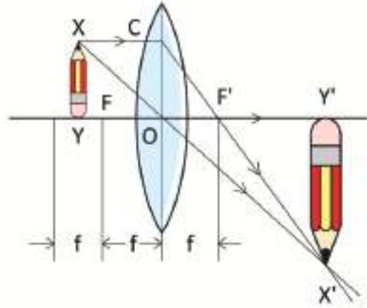
চিত্র ৯.২৪: ফোকাস দূরত্বের বাইরে কিন্তু দ্বিগুণ ফোকাস দূরত্বের ভেতরে বস্তু রাখা হলে তার বাস্তব, উল্টো ও বড় প্রতিবিম্ব তৈরি হয়।
