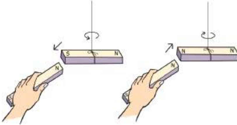
চিত্র ১২.০১: চুম্বকের বিপরীত মেরুতে আকর্ষণ ও সমমেরুতে বিকর্ষণ হয়।
