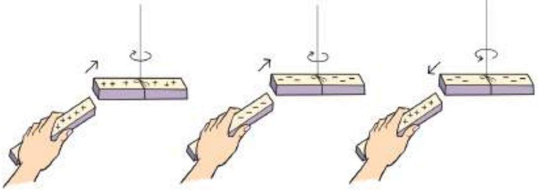
চিত্র ১০.০৩: একই ধরনের চার্জ বিকর্ষণ করে এবং বিপরীত ধরনের চার্জ আকর্ষণ করে।
