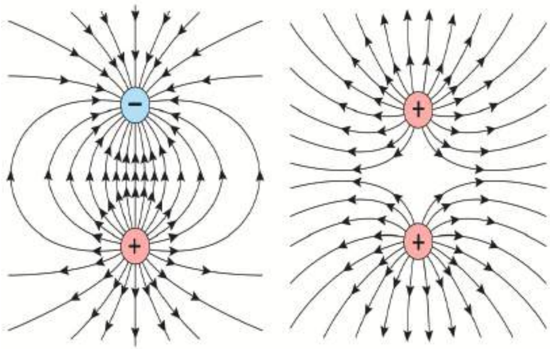
চিত্র ১০.১২: (a) বিপরীত এবং (b) সমচার্জের জন্য তৈরি বলরেখা।
