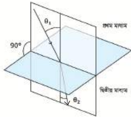
চিত্র ৯.০১: প্রথম মাধ্যম থেকে দ্বিতীয় মাধ্যমে আলোর প্রতিসরণ।
