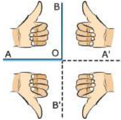
চিত্র চ.১৫: সমকোণে রাখা দুটি আয়নায় বাম হাতের মুঠির ভিন্ন ভিন্ন প্রতিফলন।
