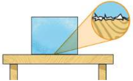
চিত্র ৩.১৬: ঘর্ষণ প্রকৃতপক্ষে দুটো এবড়োথেবড়ো পৃষ্ঠের কারণে তৈরি হয়।
