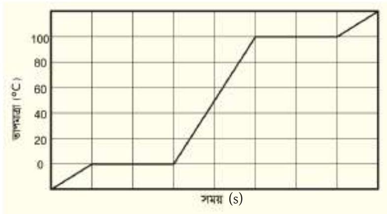
চিত্র ৬.০৮: তাপ প্রয়োগ করার সময় গলনাঙ্ক এবং স্ফুটনাঙ্কের তাপমাত্রার পরিবর্তন হয় না।
