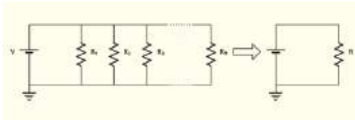
চিত্র ১১.১৪: অনেকগুলো সমান্তরাল রোধ বা রেজিস্টরকে একটি তুল্য রোধ বা রেজিস্টর হিসেবে কল্পনা করা যায়।
